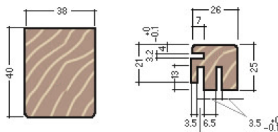
PROFILO PORTA IN LEGNO CON MURATURA 125 mm.
