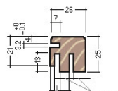
PROFILO PORTA IN LEGNO CON MURATURA 125 mm.
