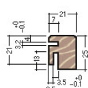
PROFILO PORTA IN LEGNO CON MURATURA 110 mm.
