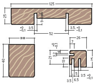
PROFILO PORTA IN LEGNO CON MURATURA 125 mm.
